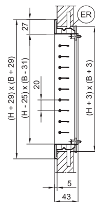
Einbauöffnung ohne Einbaurahmen (H - 10 mm) x (B - 10 mm)
