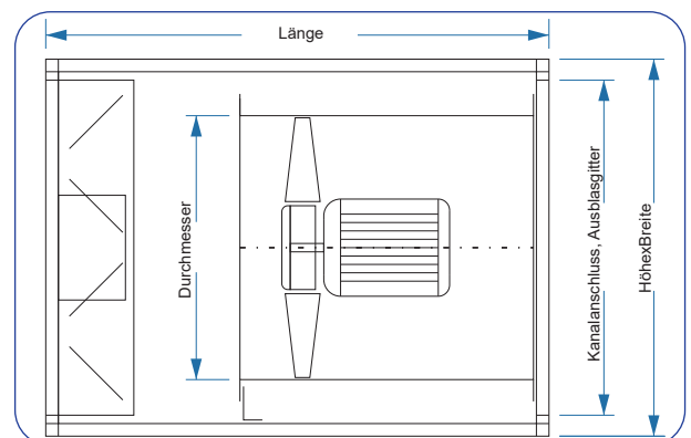
Ventilatorbox, aussen
