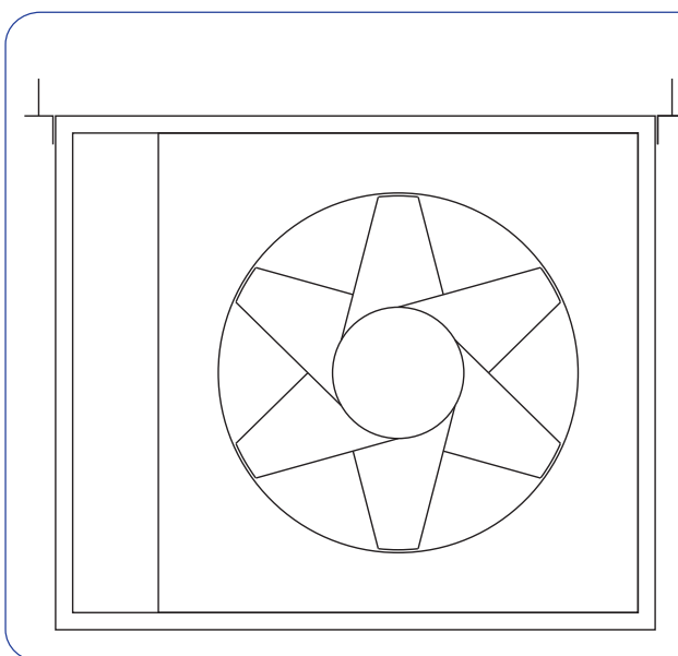
Innenansicht DBA Ventilatorbox
